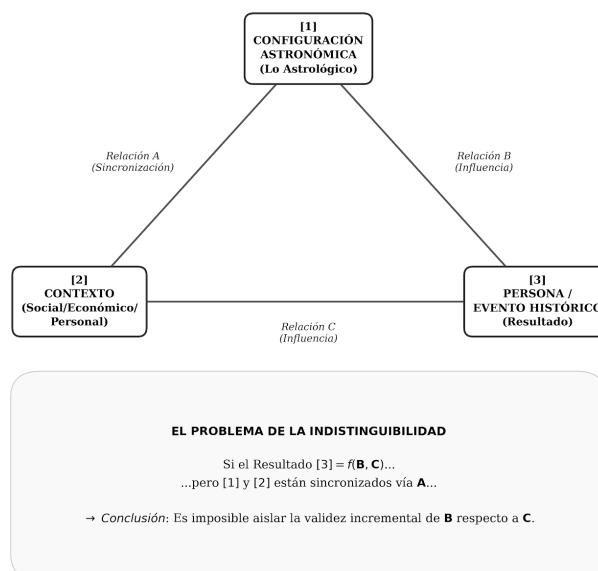
DIAGRAMA 1: EL TRIÁNGULO DE INDISTINGUIBILIDAD
